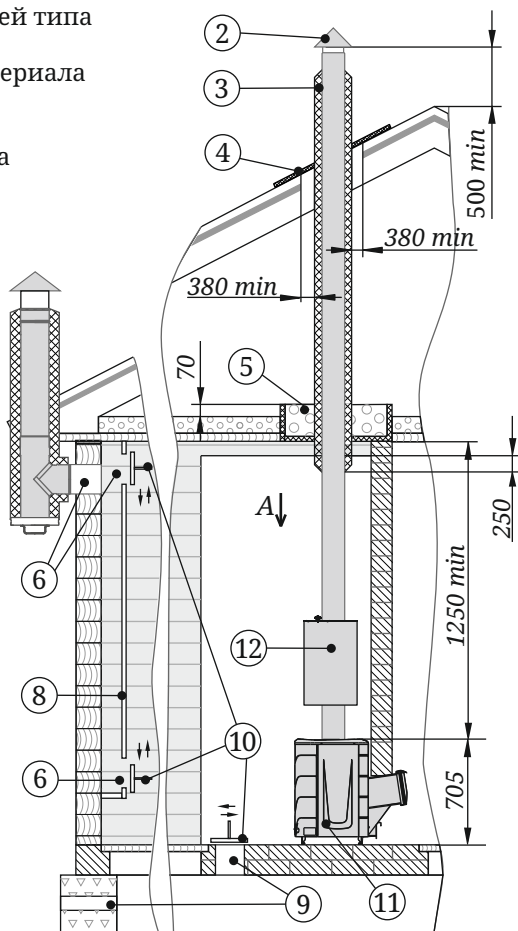
Рисунок 4. Схема монтажа печи
