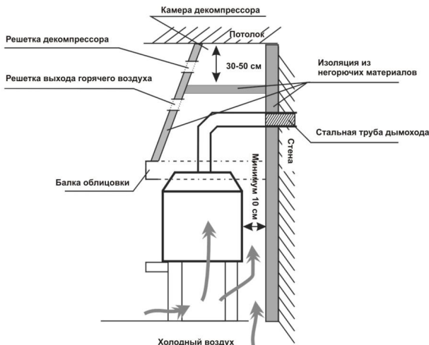
РИСУНОК 4: ВИД СБОКУ
