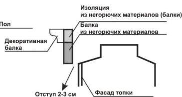
РИСУНОК 2: ОТСТУП
