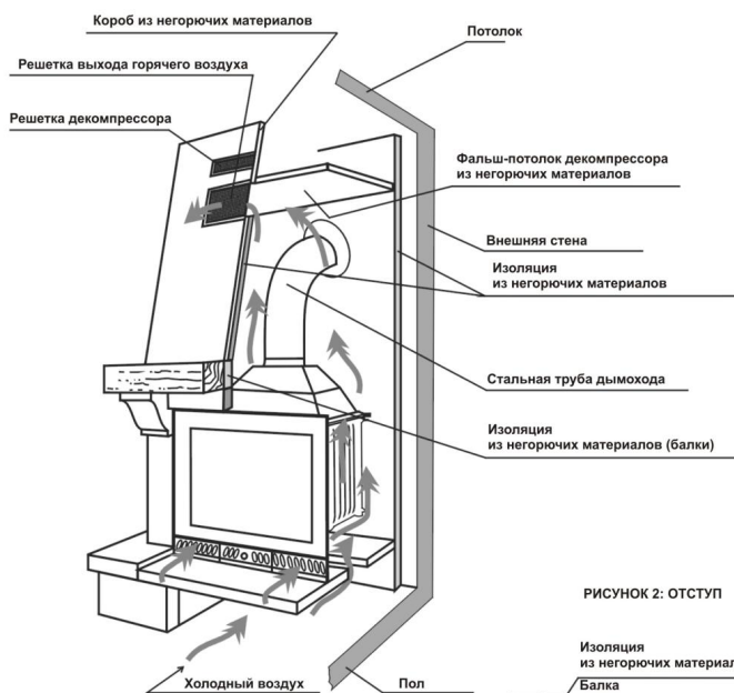
РИСУНОК 1: ПРИМЕРНЫЙ СПОСОБ УСТАНОВКИ КАМИННОЙ ТОПКИ
